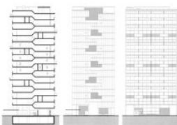
9. J. B. Bakema & J. H. van den Broek / Hansaviertel Tower, Berlin, 1957
