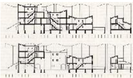
23. Gino Valle / Complesso residenziale alla Giudecca, Venezia, 1984-86
