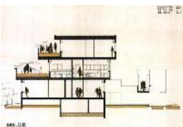
16. Giancarlo De Carlo / Villaggio Matteotti, Terni, 1969-1974
